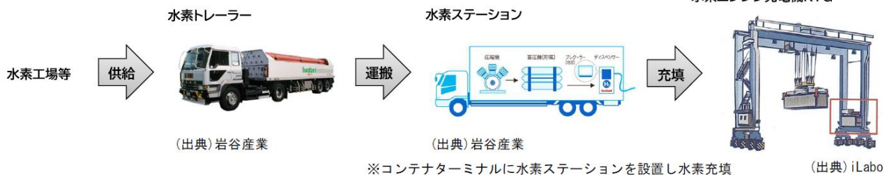
<実証事業における タイヤ式門型クレーンの水素エンジン換装(上)、水素の供給・充填(下) イメージ図>
